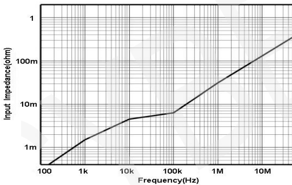
图 6 HCPX8050 输入阻抗 VS 频率曲线
