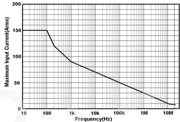
图 11.b HCPX8150A 最大测量电流 VS 频率曲线 (超过该曲线所示最大电流连续使用会导致探头烧毁)
